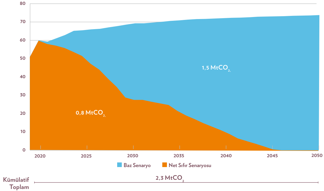
Şekil 8.2. Baz senaryoda ve Net Sıfır Senaryosunda karşılaştırmalı olarak binalardan kaynaklanan CO 2 emisyonları (MtCO 2 )
